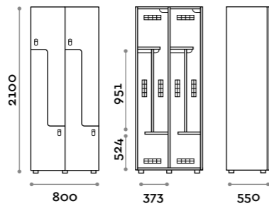
TANB49-23 Doppia colonna 4 ante a "L" Double column locker, 4 L-shaped doors
