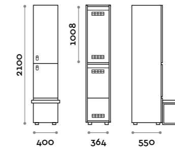
TSANB44-23 Doppia colonna 2 ante per panca a sbalzo Double column 1-tierlocker, cantilevered bench version, full lenght doors
