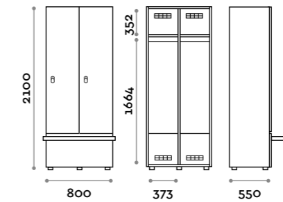
SANB44-23 Doppia colonna 2 ante per panca a sbalzo Double column 1-tierlocker, cantilevered bench version, full lenght doors
