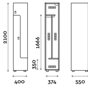
TANB49-23 Doppia colonna 4 ante a "L" Double column locker, 4 L-shaped doors
