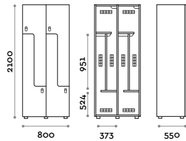
ANB49-23 Doppia colonna 4 ante a "L" Double column locker, 4 L-shaped doors
