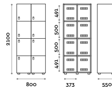
ANB428-23 Doppia colonna 8 ante Double column 4-tiers locker 8 doors
