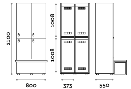
ANB45-23 Doppia colonna 4 ante per panca Double column 2-tiers locker, bench- version, 4 doors
